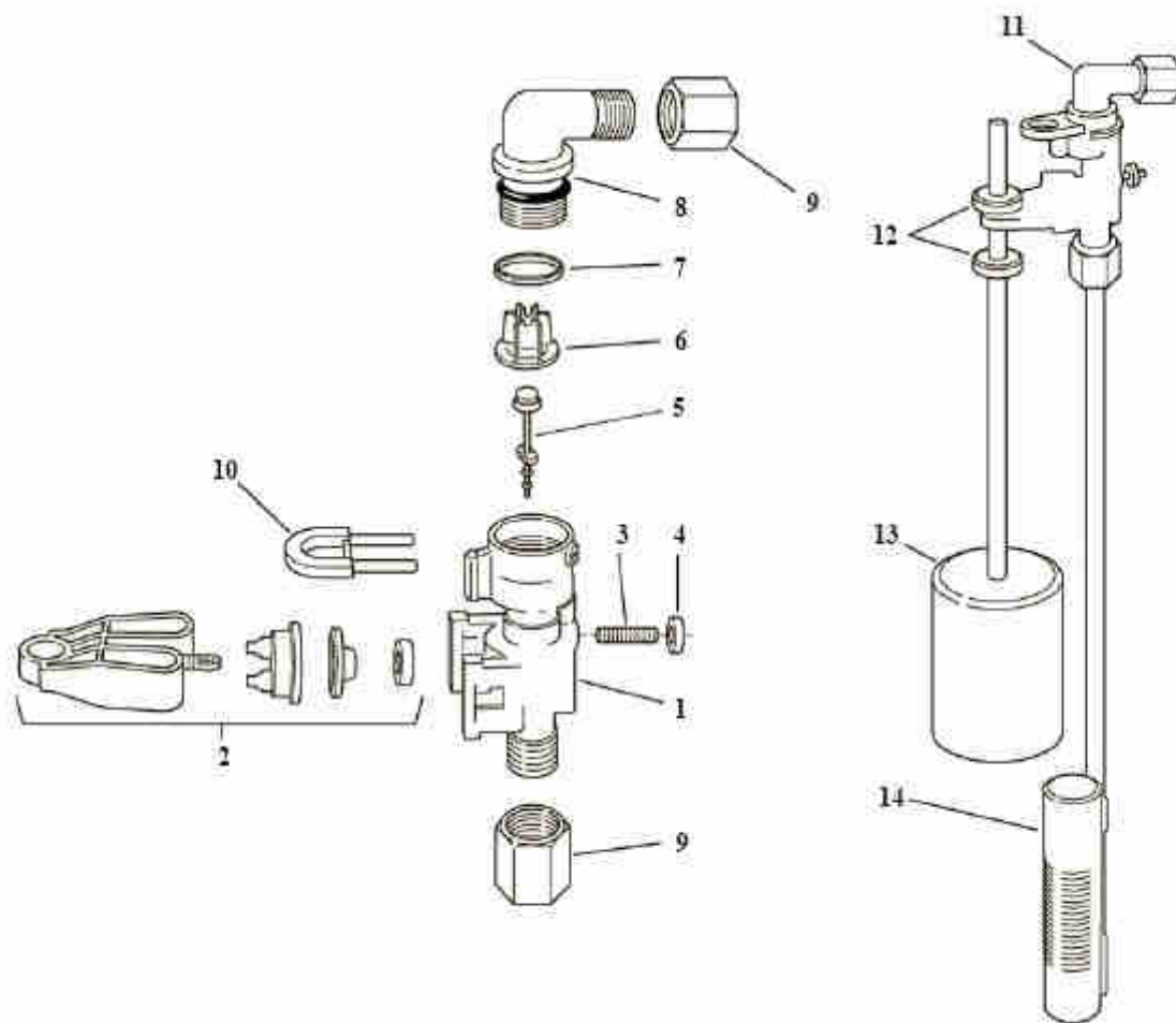
Рис. 21: Предохранительный рассольный клапан 2310
